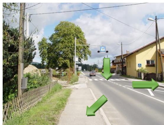
Prehod za pešce čez Mariborsko cesto v bližini osnovne šole Franca Lešnika - Vuka. Prehod je opremljen s talno svetlikajočo signalizacijo, znakom za prehod za pešce ter utripajočim semaforjem.
